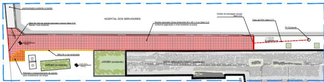
11 PLANTA DE URBANISMO ESCALA 1:500
