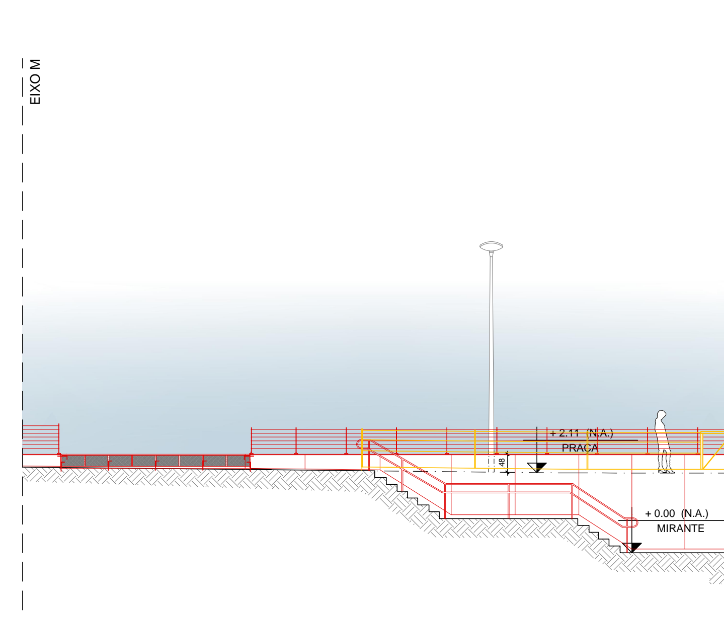
01 ELEVÇÃO A ESCALA 1:100
