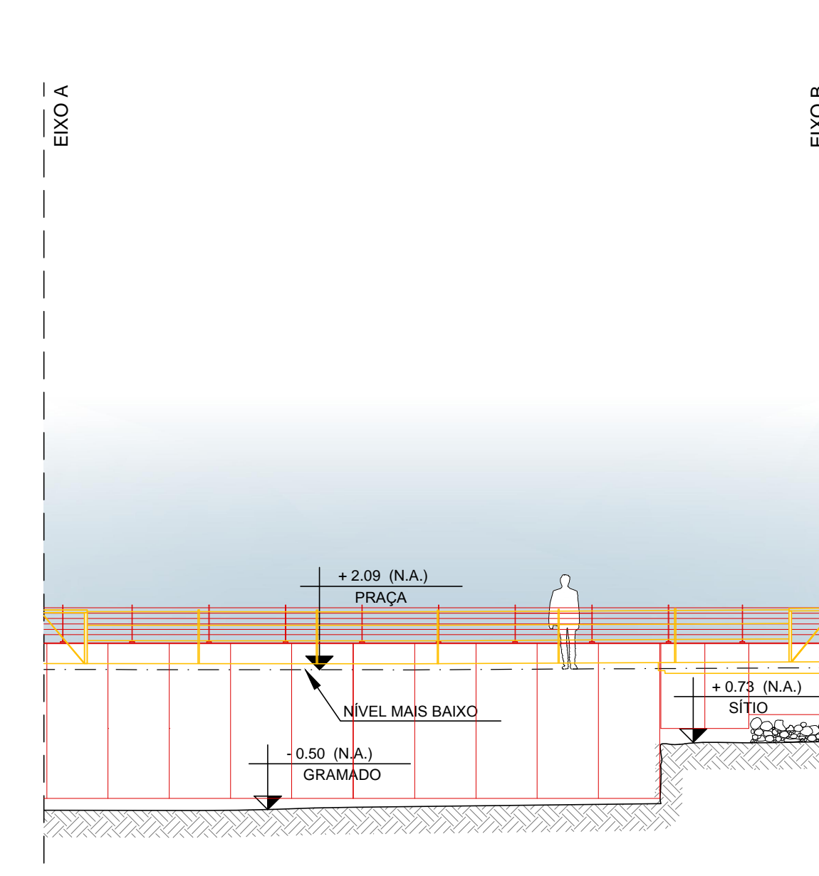
02 ELEVÇÃO B ESCALA 1:100
