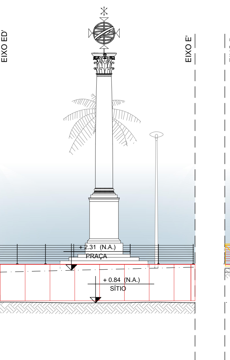
04 ELEVÇÃO E' ESCALA 1:100
