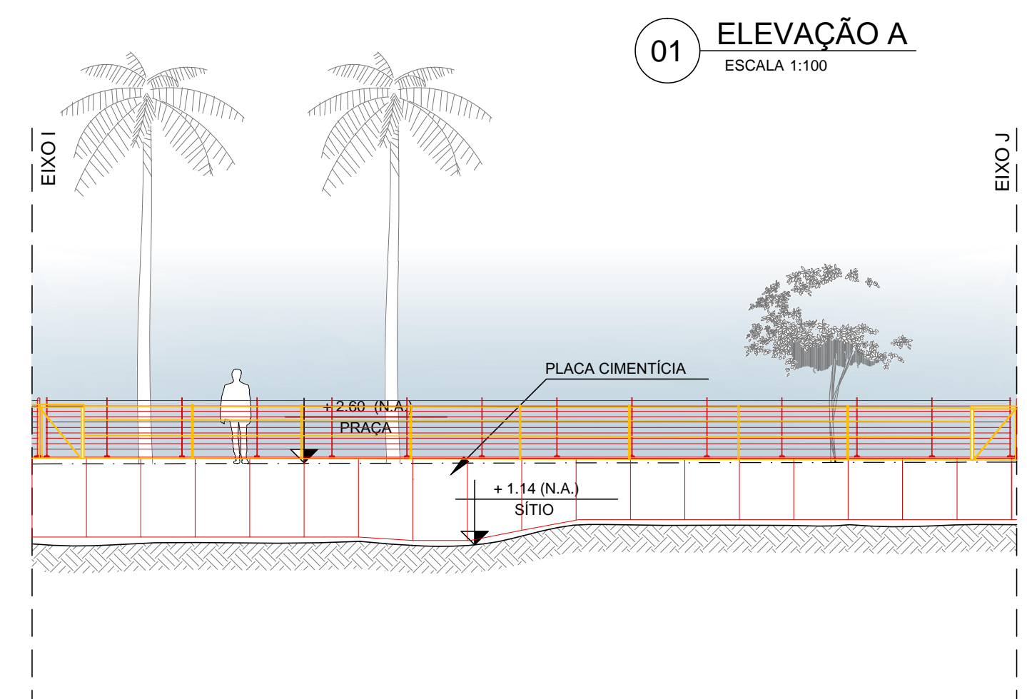
10 ELEVÇÃO J ESCALA 1:100
