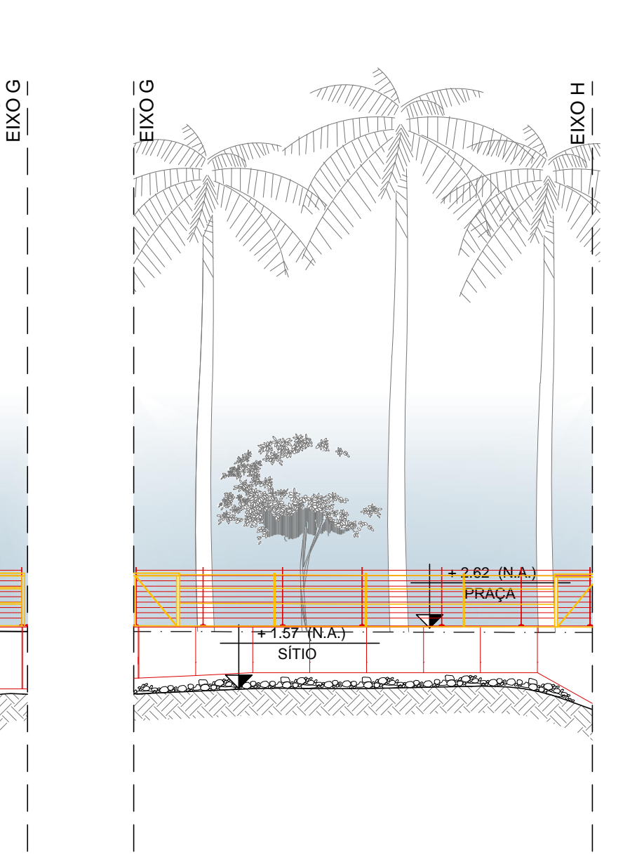
07 ELEVÇÃO G ESCALA 1:100
