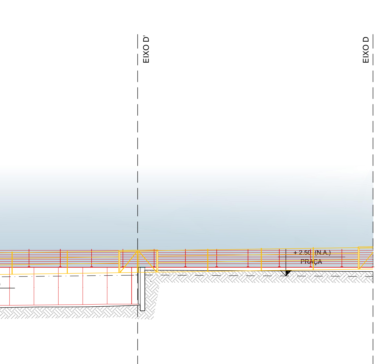
04 ELEVÇÃO D ESCALA 1:100
