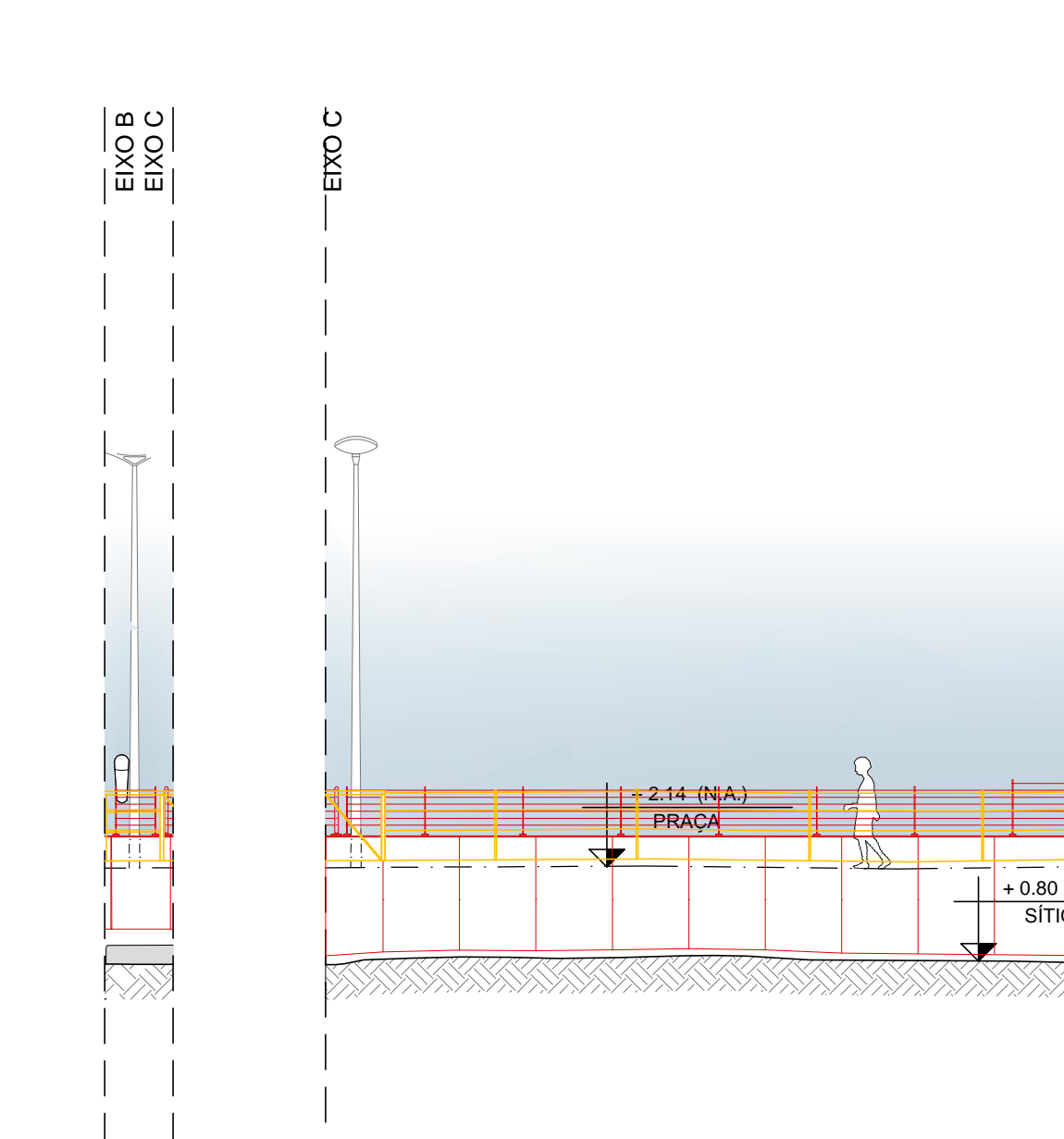
03 ELEVÇÃO C ESCALA 1:100
