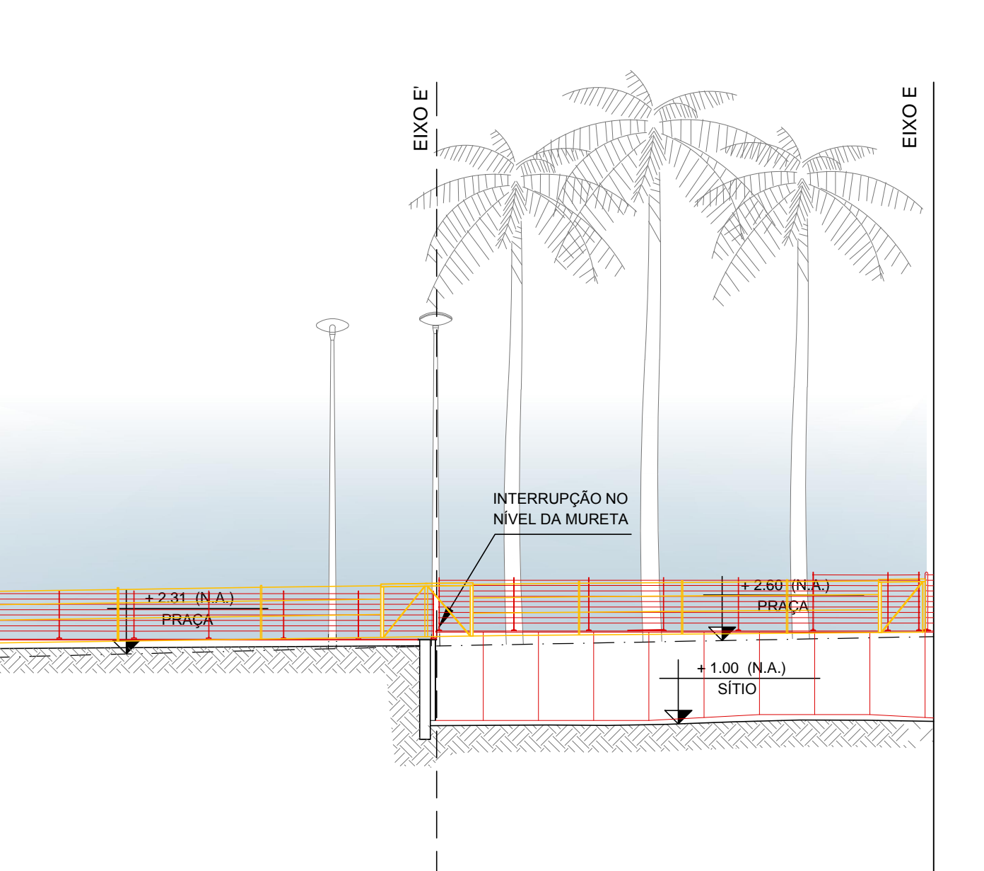
06 ELEVÇÃO F ESCALA 1:100
