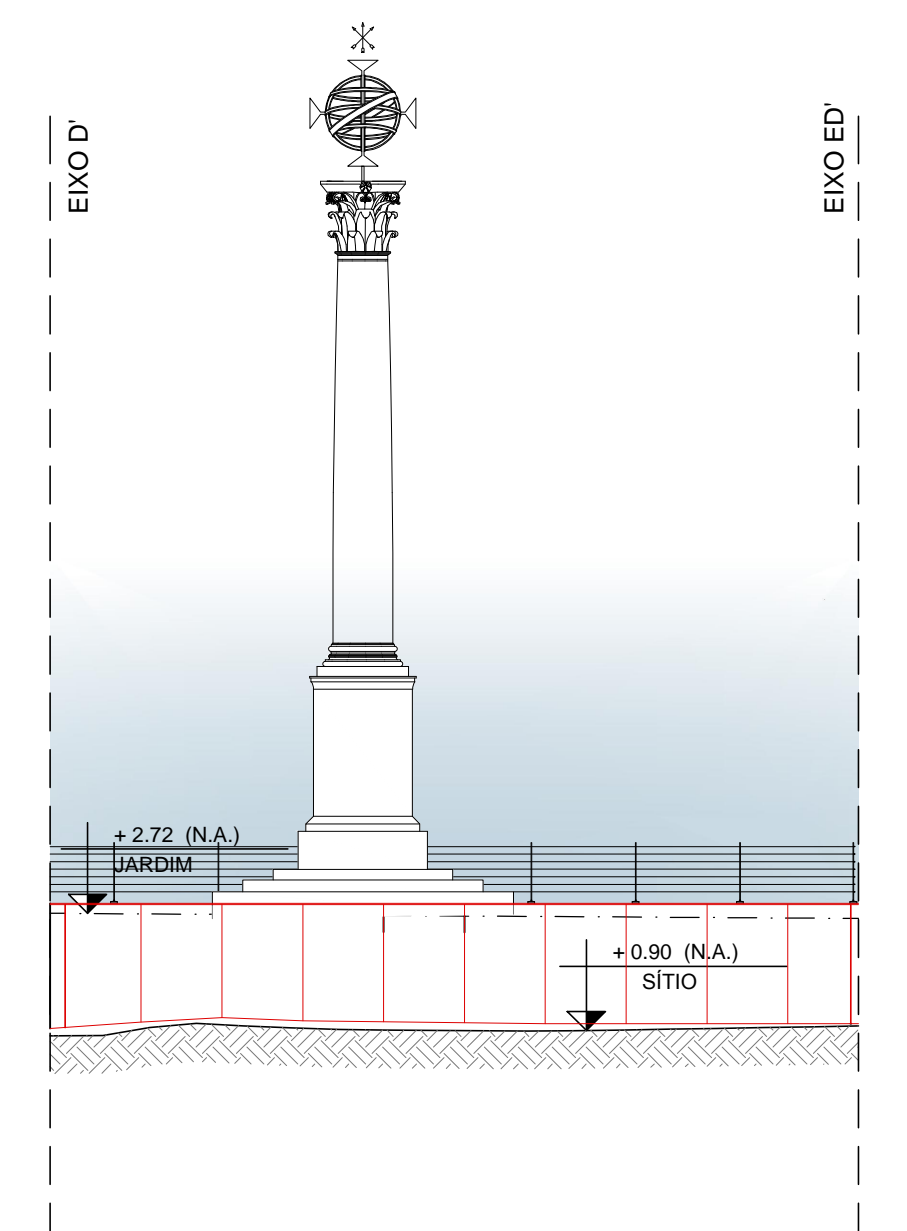
04 ELEVÇÃO D' ESCALA 1:100
